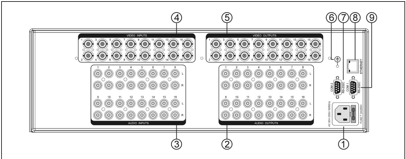
图 3.6 TMX-08xxAV 及 TMX-16xxAV 机型后面板示意图 (以 TMX-1616AV 为例)
