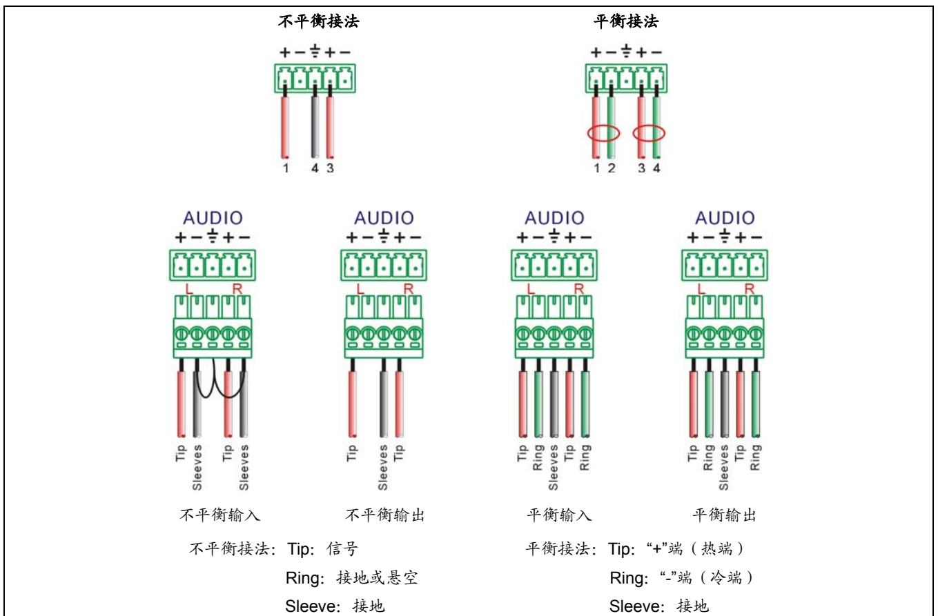
图 3.13 平衡接法与不平衡接法
