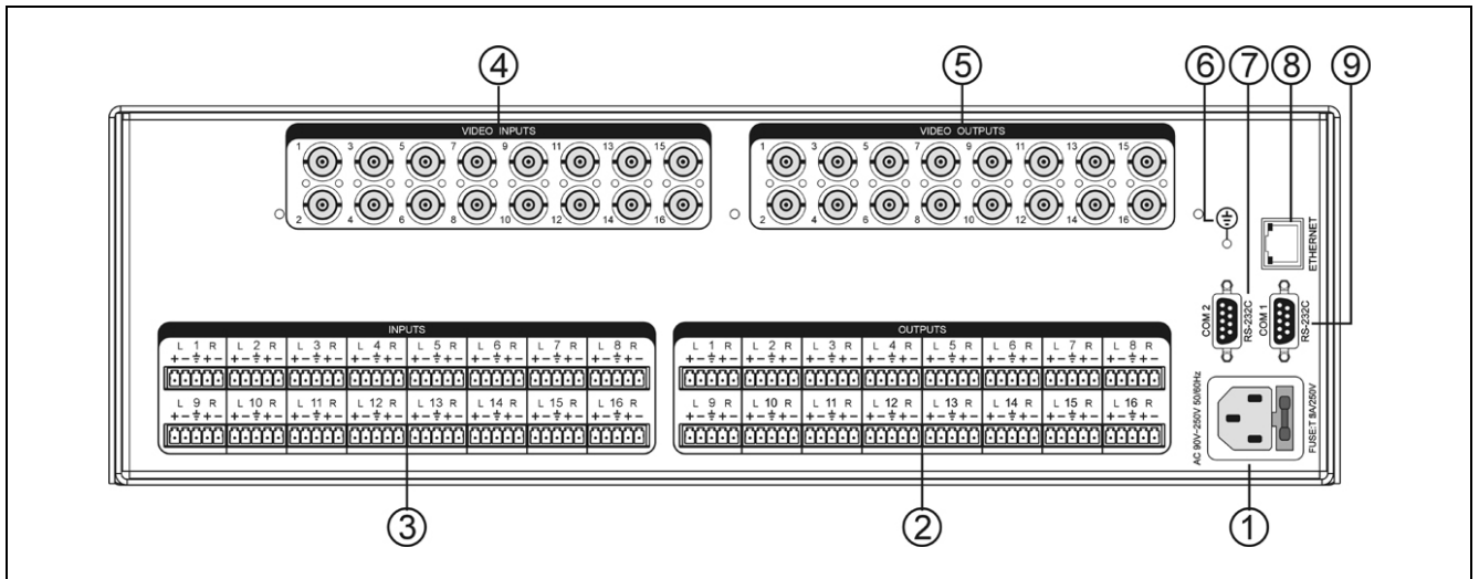
图 3.7 TMX-08xxAV-B 及 TMX-16xxAV-B 后面板示意图 (以 TMX-1616AV-B 为例)
