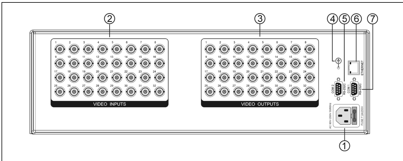
图 3.9 TMX-32xxV 后面板示意图
