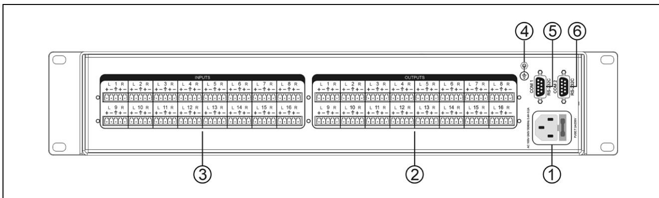
图 3.8 TMX-16xxA-B 后面板示意图
