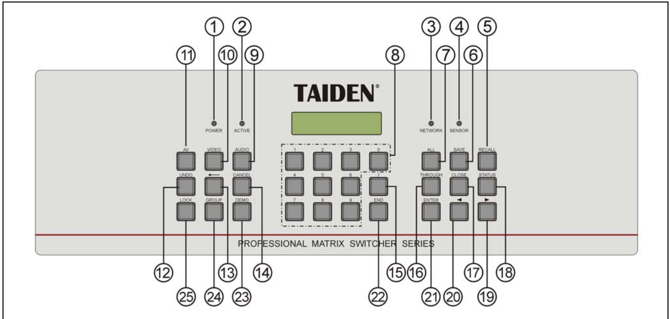
图 3.3 TMX-08xxAV(-B)、TMX-16xxAV(-B)、TMX-32xxV/AV-B 及 TMX-6464AV-B 机型前面板示意图
