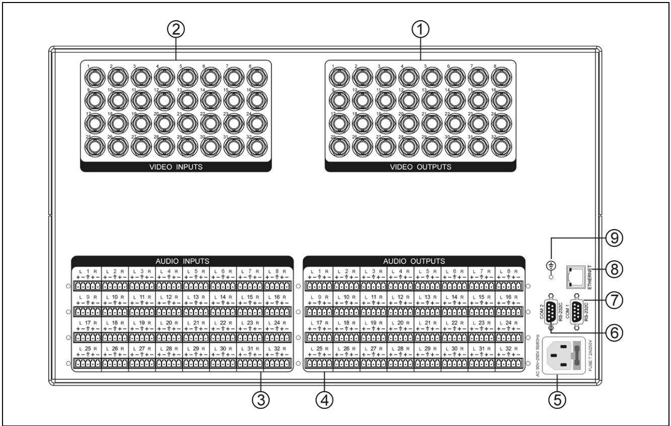
图 3.10 TMX-32xxAV-B 机型后面板示意图
